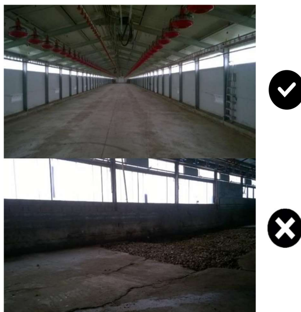
Figura 10 - Caratteristiche strutturali idonee (in alto) e non idonee (in basso) a causa della presenza di numerose crepe sul pavimento
